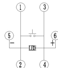
电原理图
