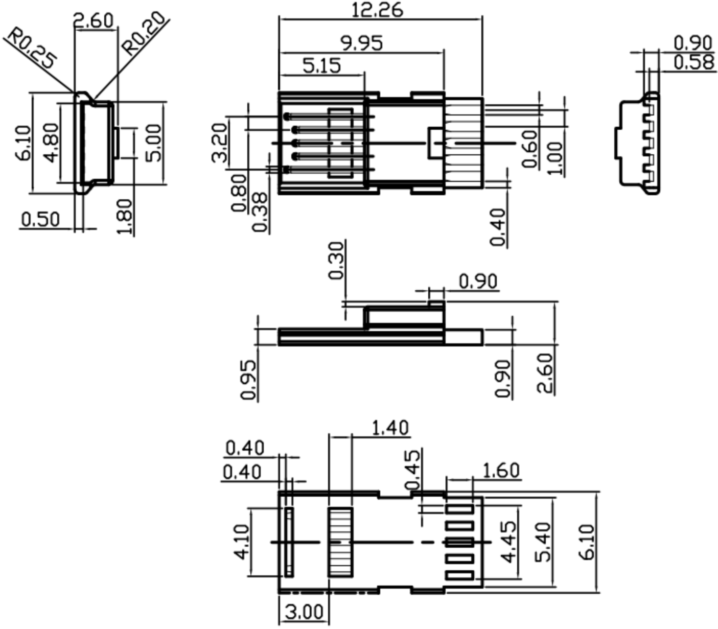
MiniUSB 5P(M) 膠芯+端子
