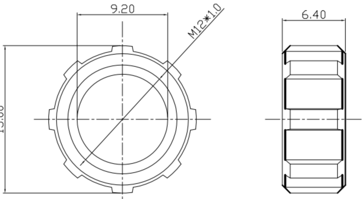
防水MiniUSB 螺母
