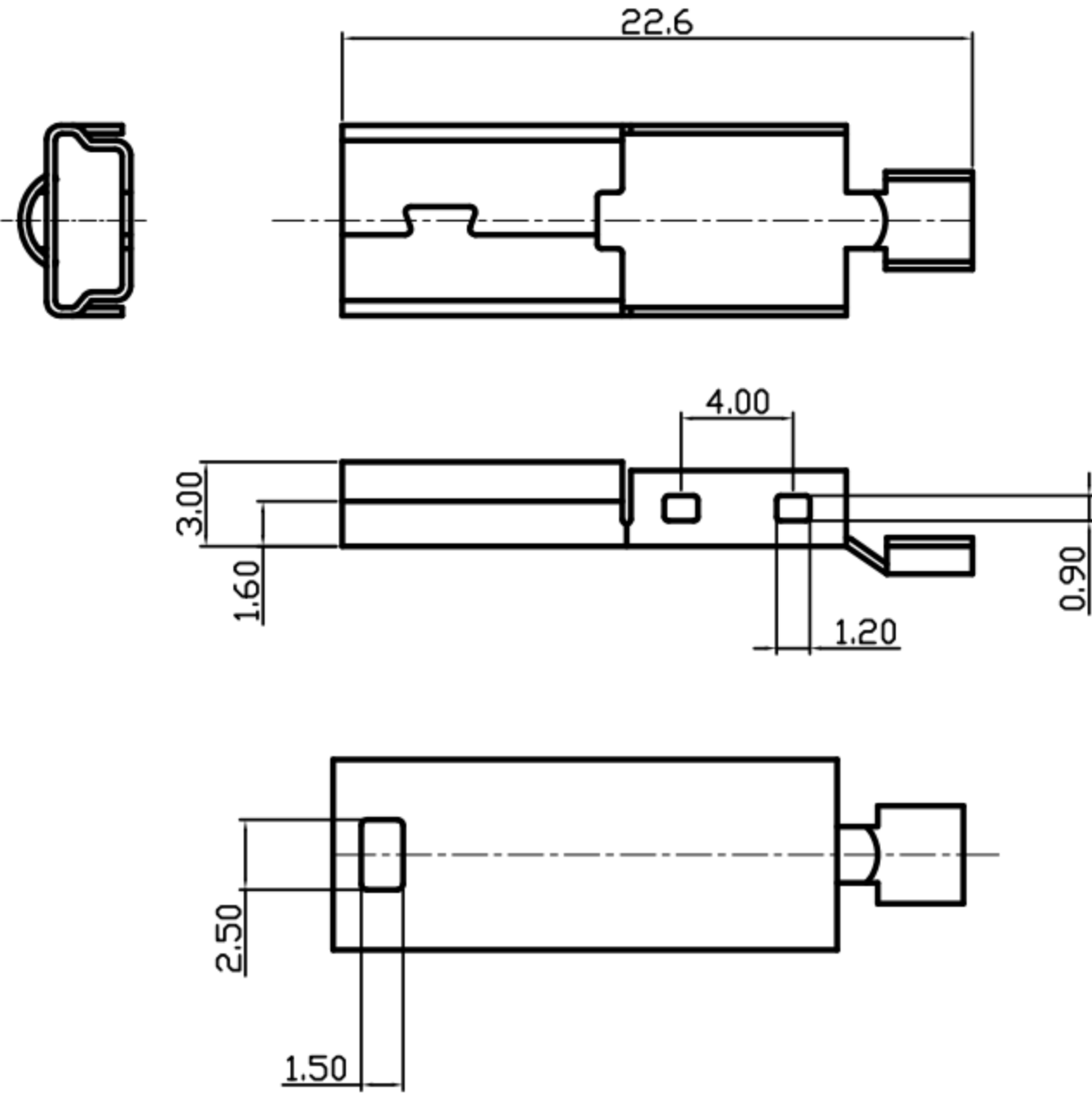
MiniUSB 5P(M) 成型下蓋
