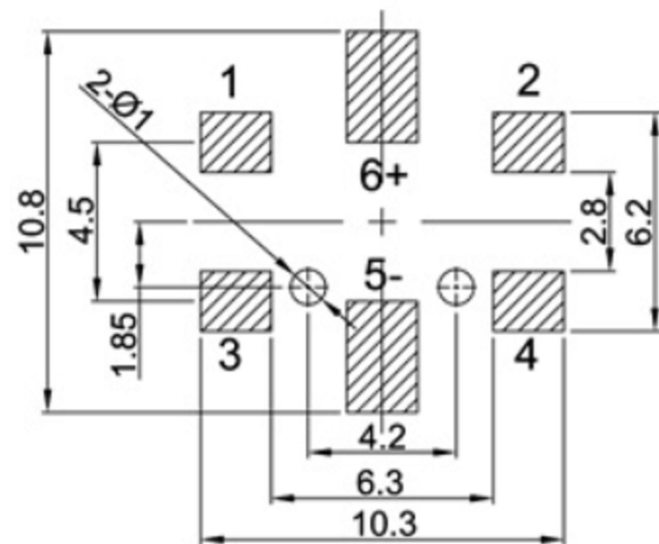
P.C.B. LAYOUT
