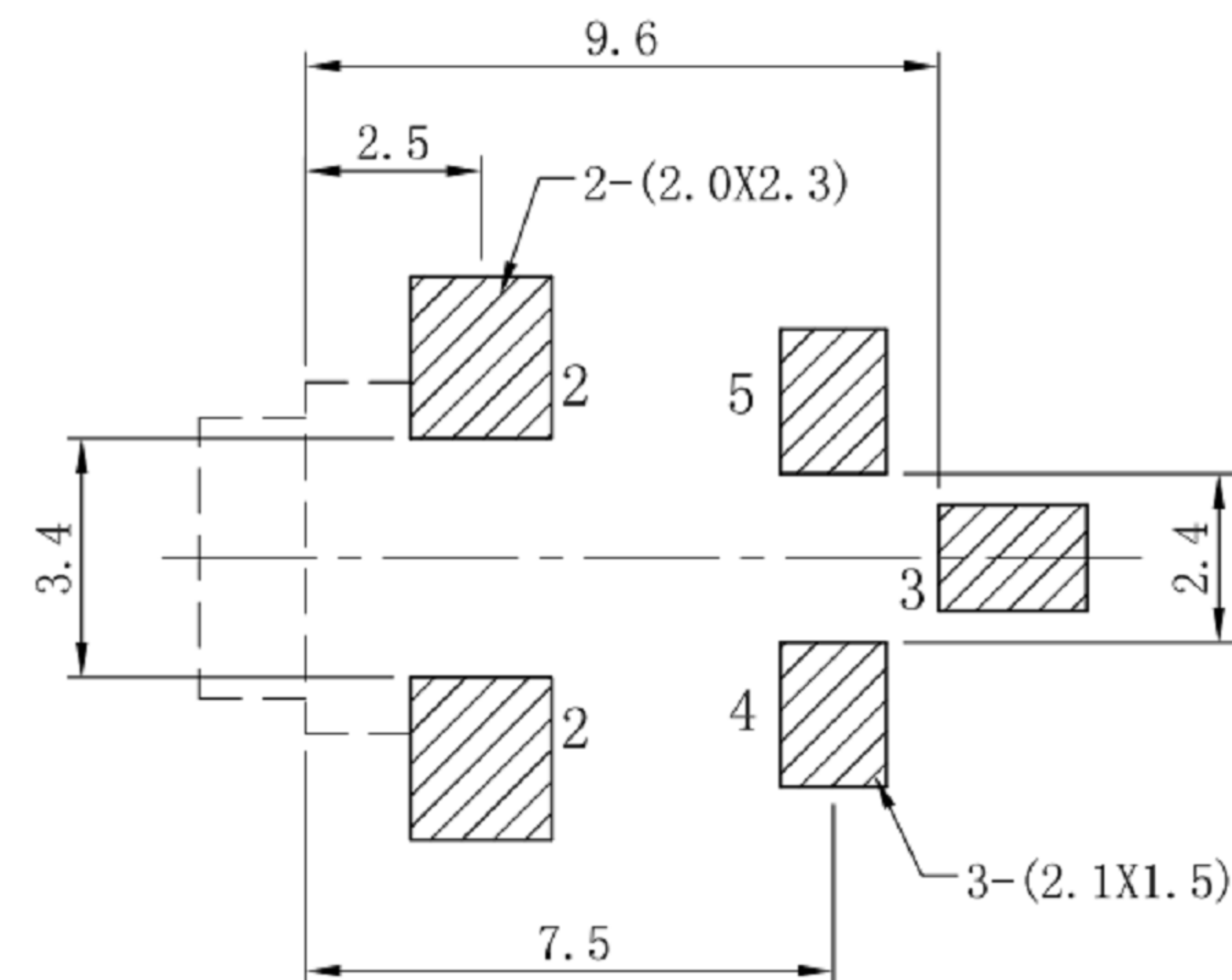
线路板开孔尺寸 P.C.B LAYOUT
