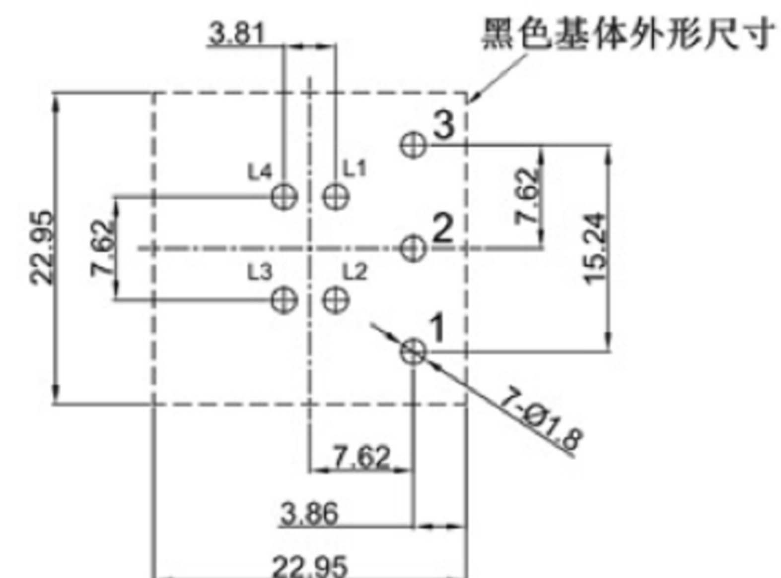
P. C. B. LAYOUT
