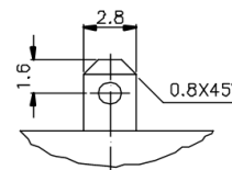
A DETAIL 4 : 1
