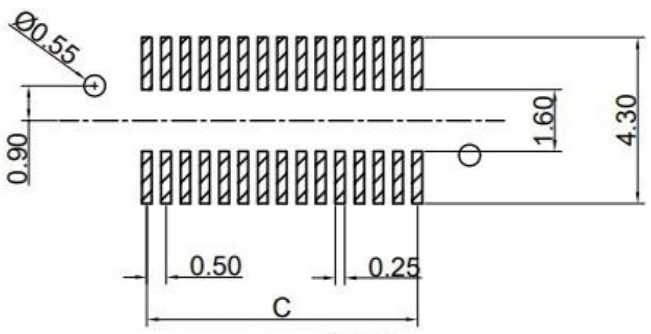
PCB 寸法
