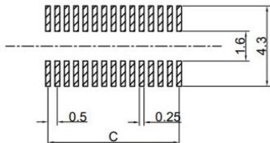
PCB 寸法
