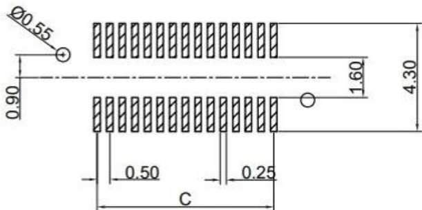
PCB 寸法
