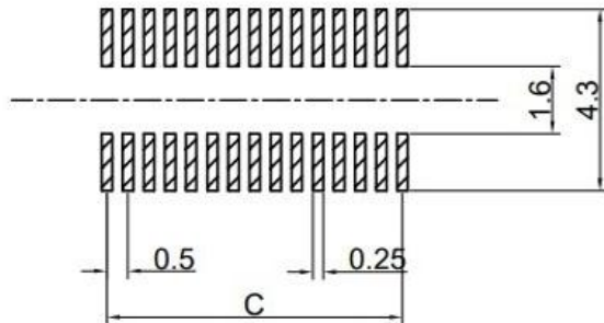
PCB 寸法
