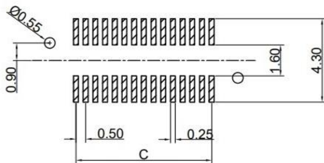
PCB 寸法
