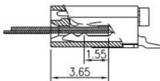
CABLE INSERT DIM.
