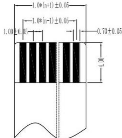
适用扁平电缆
