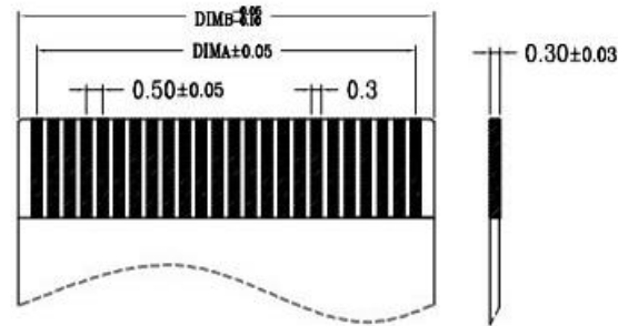
适用扁平线
