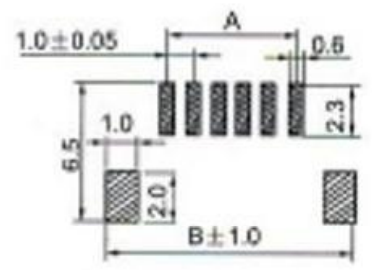
印制线路板 PCB P.C.B Layout
