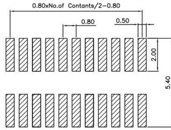
P.C.B Layout(Top Side)
