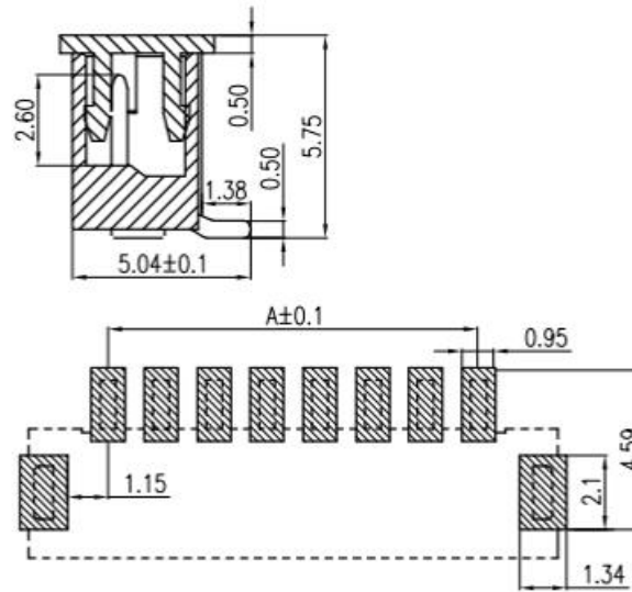
截面 A-A
