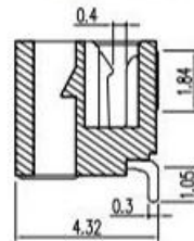
截面 A-A
