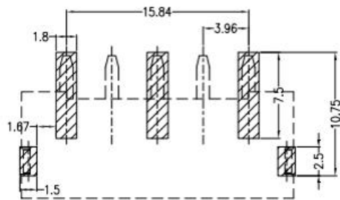
Mating PE detail
