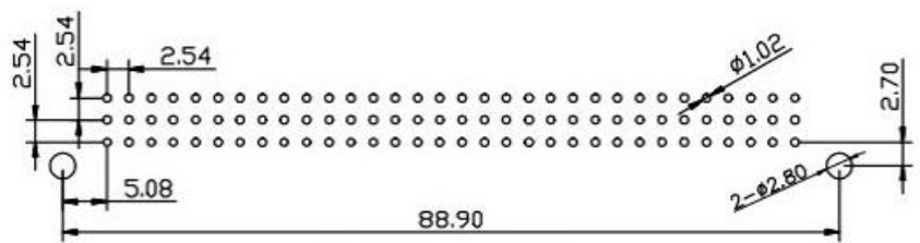
P.C.B LAYOUT
