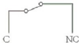
电路简图
