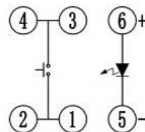
电原理图
