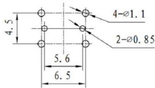
P. C. B. Land Pattern
