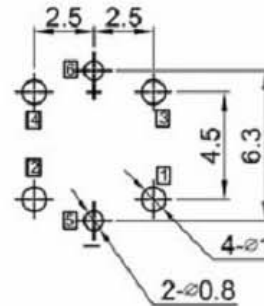
P.C.B. LAYOUT
