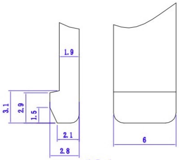
1.5: 1 锁舌参考规格
