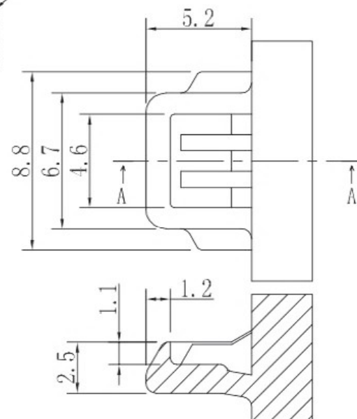
A-A 锁舌参考规格
