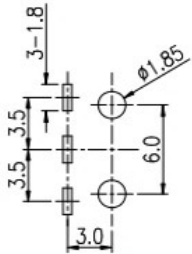
P.C.B LAYOUT
